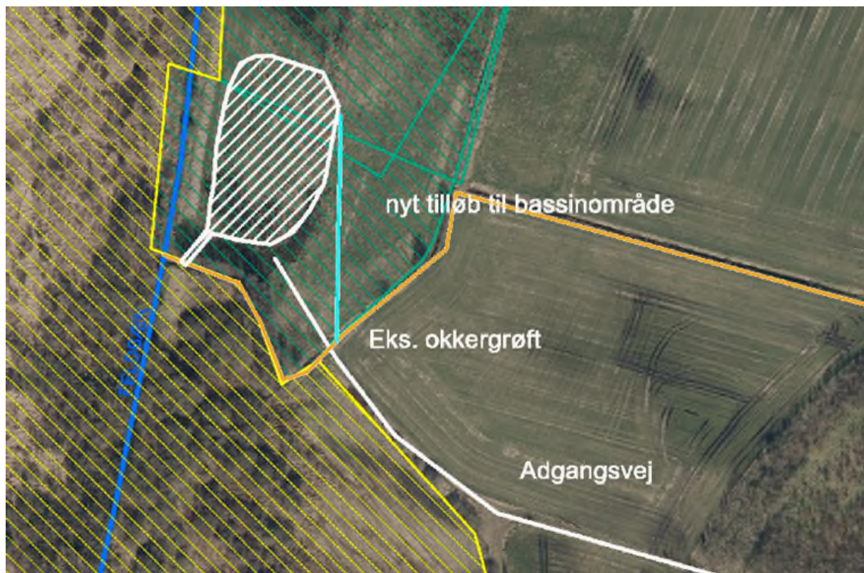
Figur 2. Projekttegning af okkerbassin. Hvid markering angiver det planlagte projektområde for bassinet. Gul markering angiver §3 eng, mens grøn markering angiver §3 eng.
