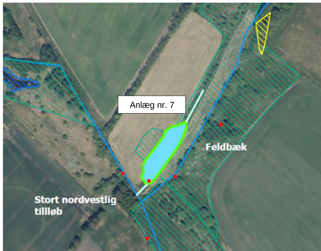
Figur 2. Projekttegning af okkerbassin. Lyseblå markering angiver det planlagte projektområde. Gul markering angiver §3 mose, mens grøn markering angiver §3 eng.
